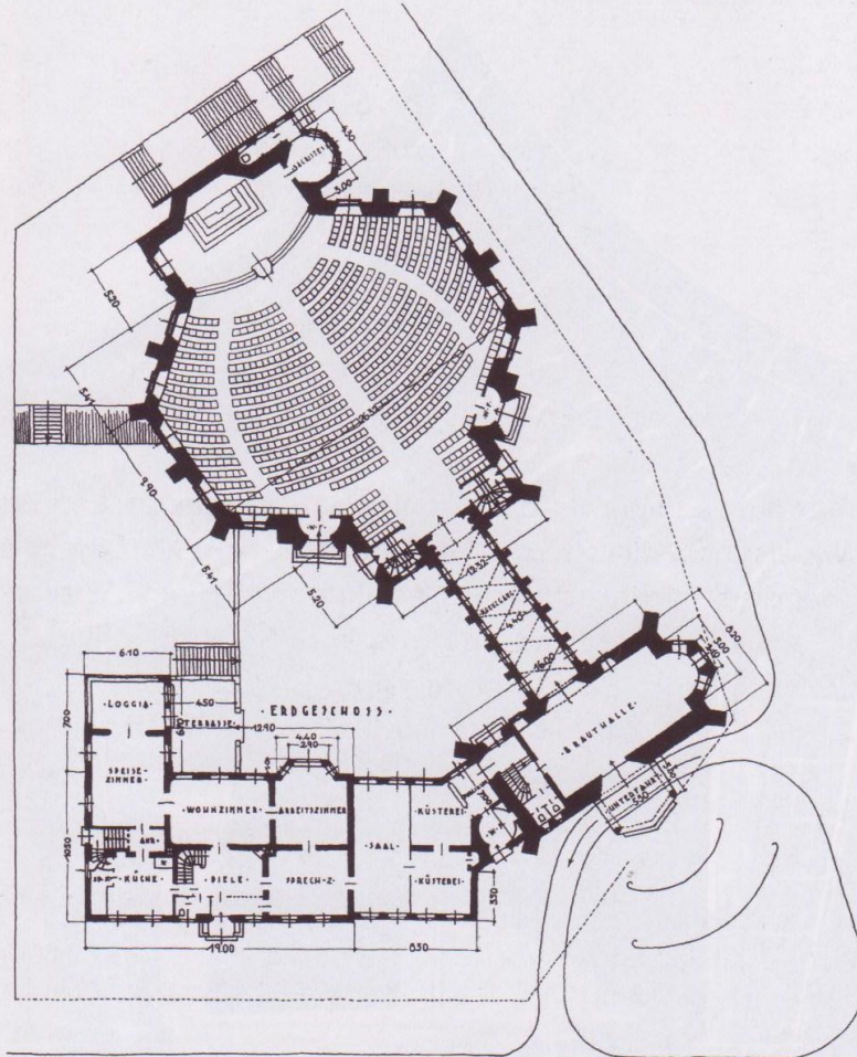
▲ Grundriss, 1930
