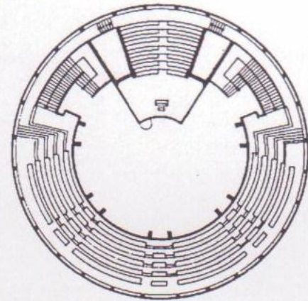
Emporengrundriß
