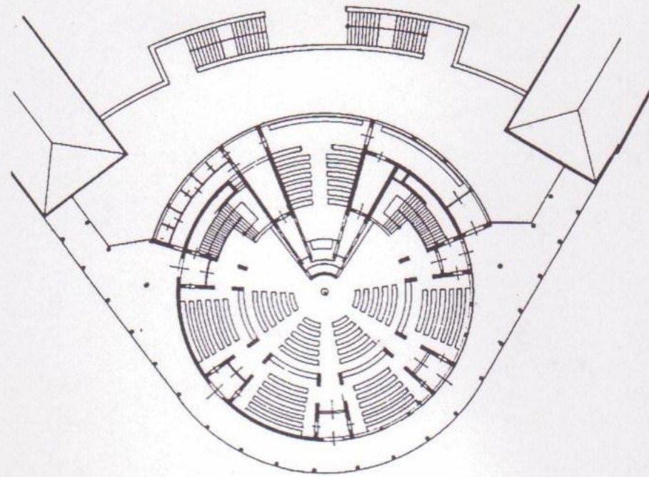
Erdgeschoßgrundriß
